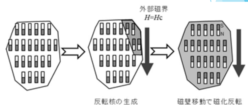
図5.14 核生成型磁性体における反転機構の模式図
