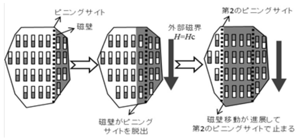
図5.15 ピニング型磁性体の反転機構の模式図
