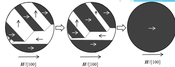
図5.11 Fe[100]方向に磁界を印加した時の磁壁移動と磁気飽和。弱い磁界で飽和磁化に達する
