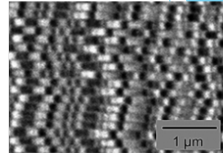
図5.1 垂直磁気記録された記録磁区のMFM像（中央大学二本先生による）
