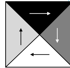
図4.12 環流磁区構造
