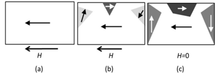
図5.16 磁気飽和状態から磁界を減らしていくと、さまざまな磁化方向の磁区が核発生し、成長するが、もとの状態には戻れない。
