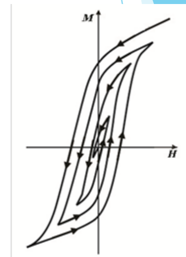
図5.8 交流消磁の消磁過程
