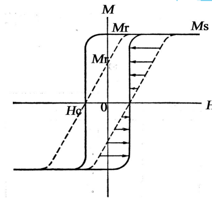
図4.7 測定した磁化曲線は図の点線のように傾いているが、磁気モーメントに加わる磁界が反磁界の分だけ減少しているため、適切な補正を行うと実線のようになる。
