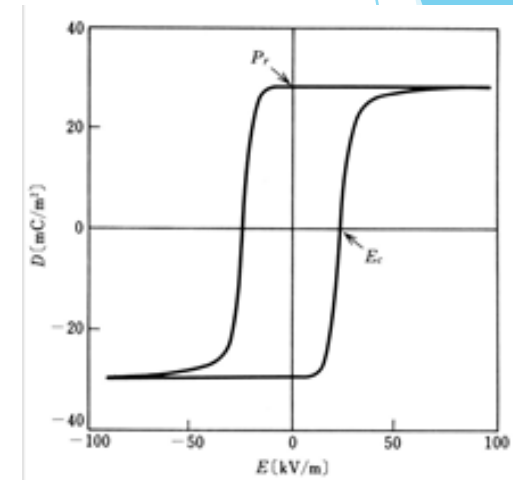
図5.4 強誘電体硫酸グリシン(TGS)の誘電ヒステリシスループ
