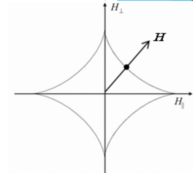
図5.17 磁化反転の臨界磁界曲線
