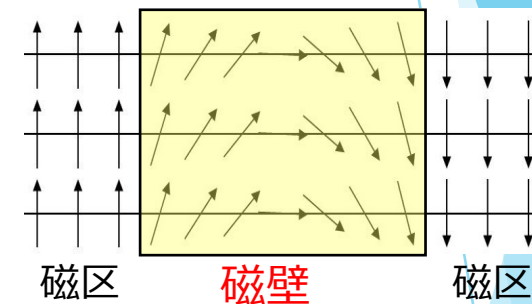
図4.11 磁壁内では原子磁石が徐々に回転して隣り合う磁区の磁化をつなぐ
