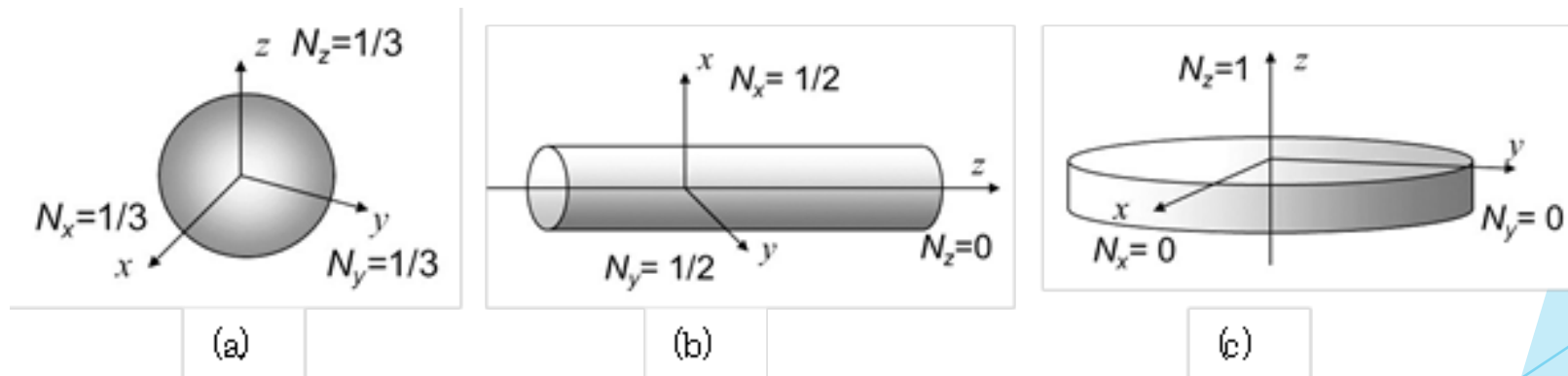
図4.6 反磁界係数は磁性体の形と向きで異なる。
