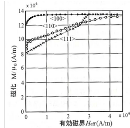
図5.9 Feの磁化曲線の結晶方位依存性(Kayaによる。佐藤勝昭編著 応用物性 p209)
