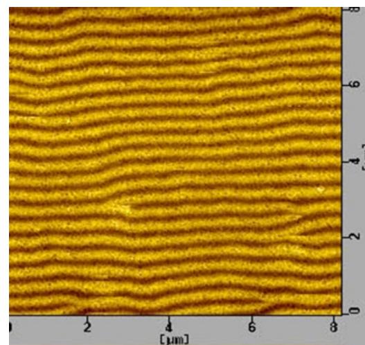
図4.10 磁気力顕微鏡(MFM)で見た縞状磁区の像
