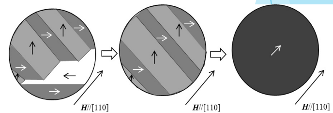
図5.12 Fe[110]方向に磁界を印加した時は、磁壁移動によって[100]磁区と[010]磁区が埋め尽くし磁化が M_s/\sqrt{2} をとった後、磁化回転が起きて飽和磁化状態に達する。
