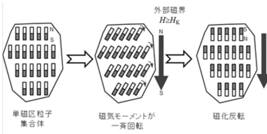
図5.13 単磁区粒子集合体における反転機構の模式図
