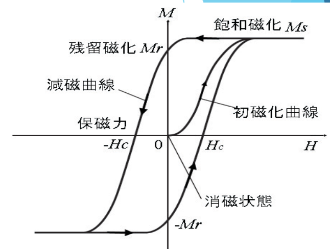
図5.3 強磁性体の典型的な磁化曲線
