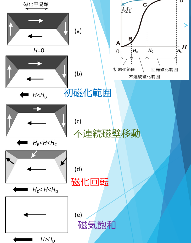
図5.7 初磁化曲線の磁壁移動・磁化回転による説明
