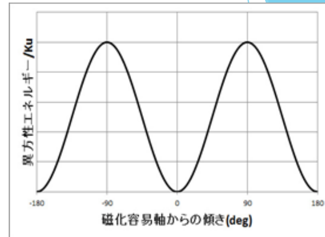
図5.10 磁化容易軸からの傾きと磁気異方性エネルギーの関係
