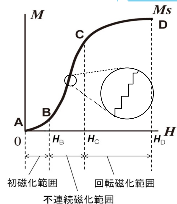
図5.6 初磁化曲線
