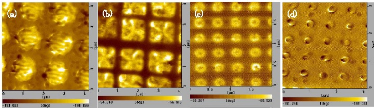
図 4.14 微細ドットの磁気構造 (a) 縞状磁区(Co 円形ドット 1.2\mu\text{m}\phi ), (b) 環流磁区(パーマロイ正方形ドット 1.2\mu\text{m} ), (c) ボルテックス(パーマロイ円形ドット 300\text{nm}\phi ), (d) 単磁区(Co 円形ドット 100\text{nm}\phi )
