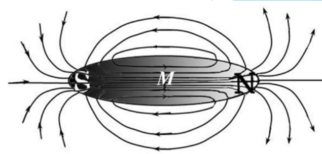
図4.4 磁束線は磁化と連続
