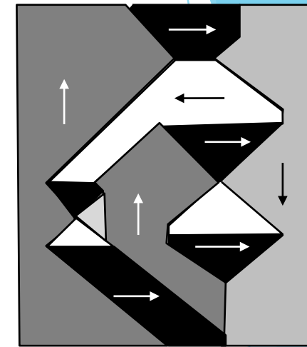
図4.2 磁化前の磁性体の磁区構造の模式図
