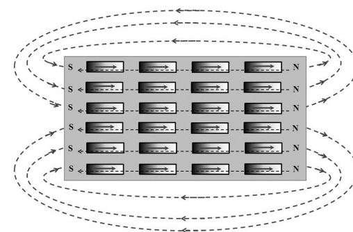
図4.8 磁性体内部の原子磁石は反磁界を受けて静磁的に不安定
