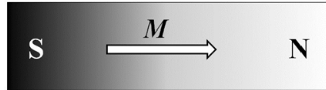
図4.3 磁性体の内部には多数の原子磁石があるが隣り合う原子磁石は打ち消しあい両端に磁極が生じる
