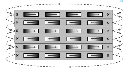
図4.9 右向きの磁化をもつ領域と左向きの磁化をもつ領域とに縞状に分かれると反磁界は打ち消しあって安定になる
