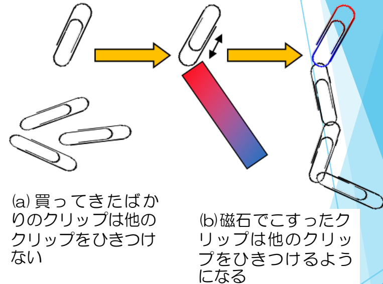
図4.1 鉄のクリップを磁石でこすると磁気を帯びる
