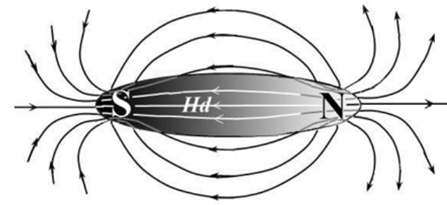
図4.5 磁力線はN極からS極に向かって流れている
