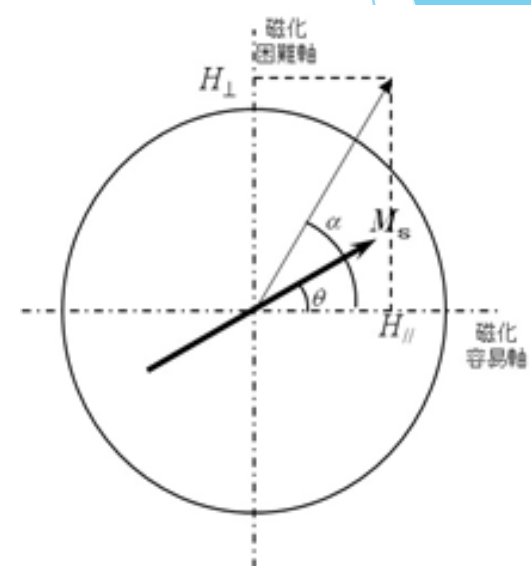
図5.19 単磁区磁性体の磁化回転メカニズムを理解するための模式図
